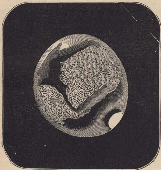
Marte en su cuarto menguante.
